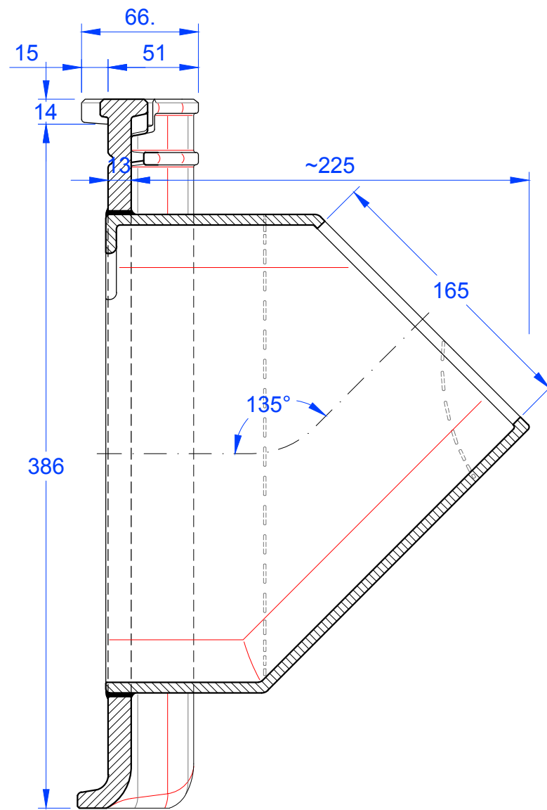
Schnitt B-B
