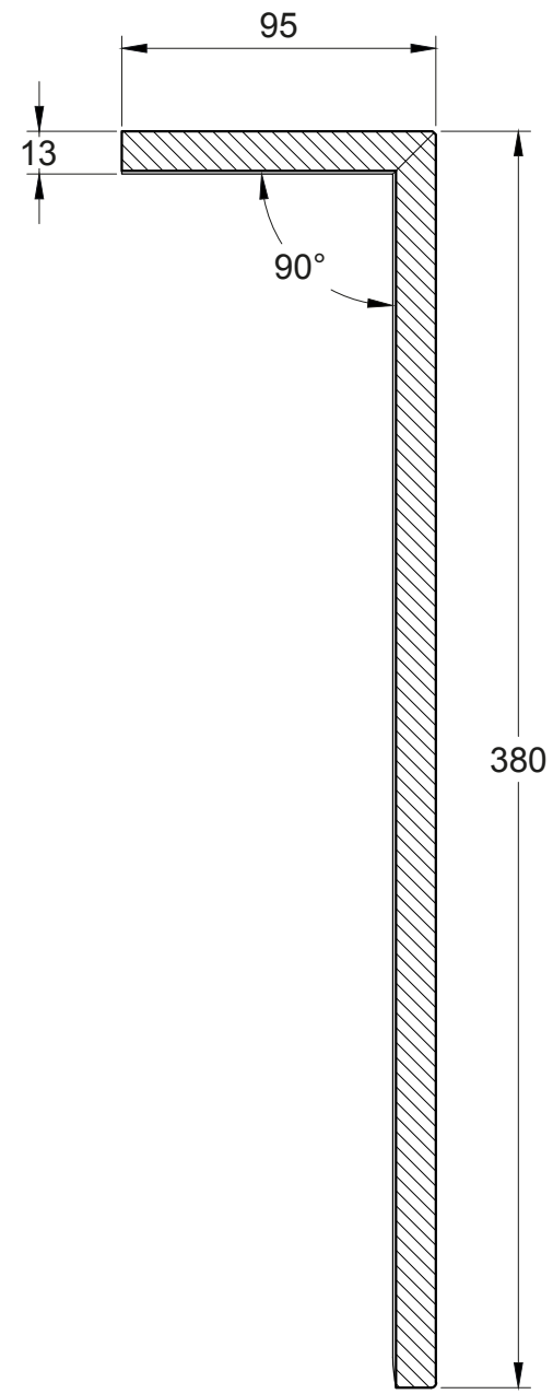
Schnitt B-B
