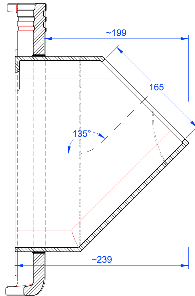
Schnitt B-B
