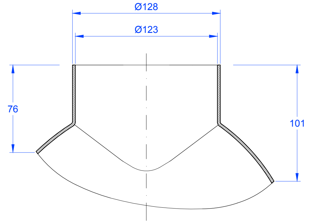
Schnitt A-A
