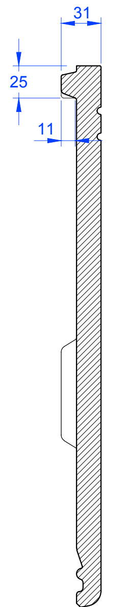
Schnitt B-B
