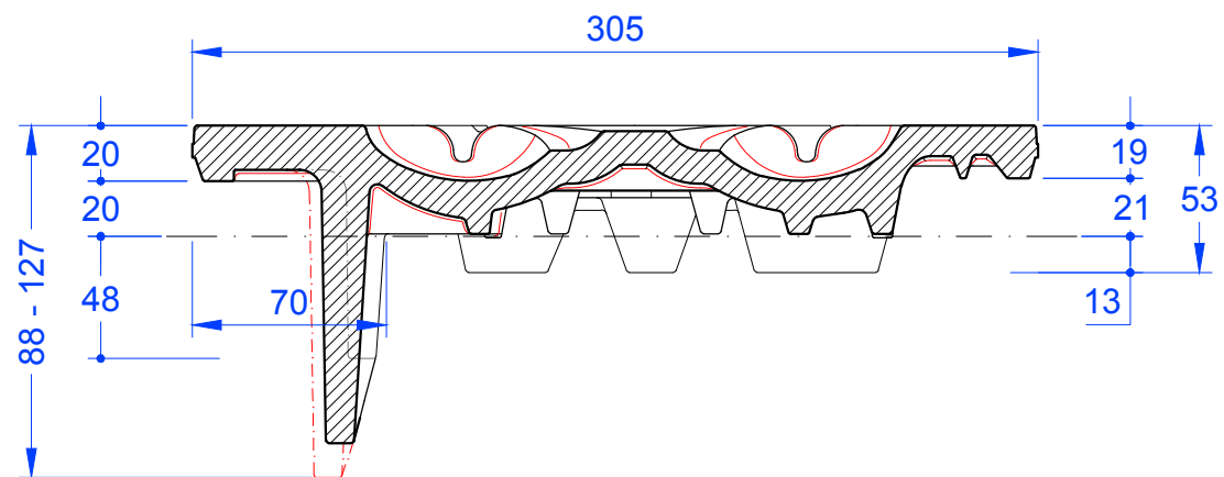
Schnitt A-A
