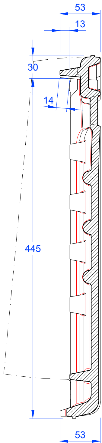
Schnitt B-B
