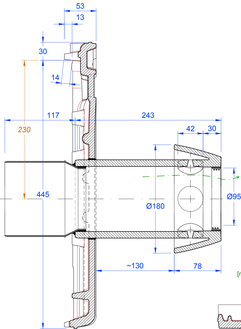
Schnitt B-B (ohne Deckel)
