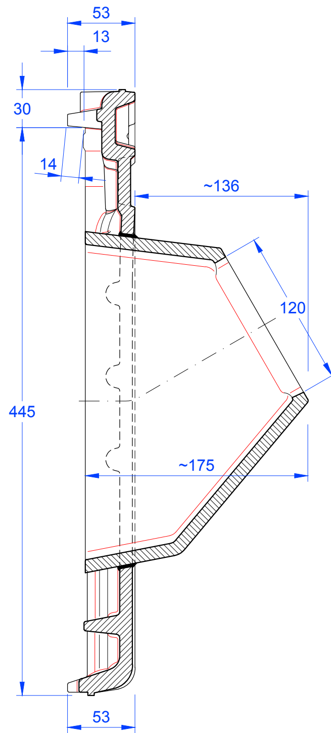
Schnitt B-B
