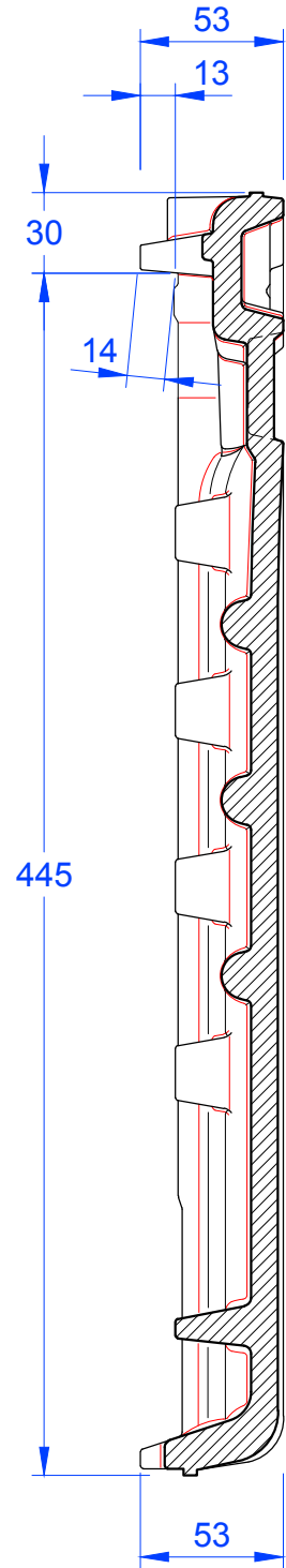
Schnitt B-B
