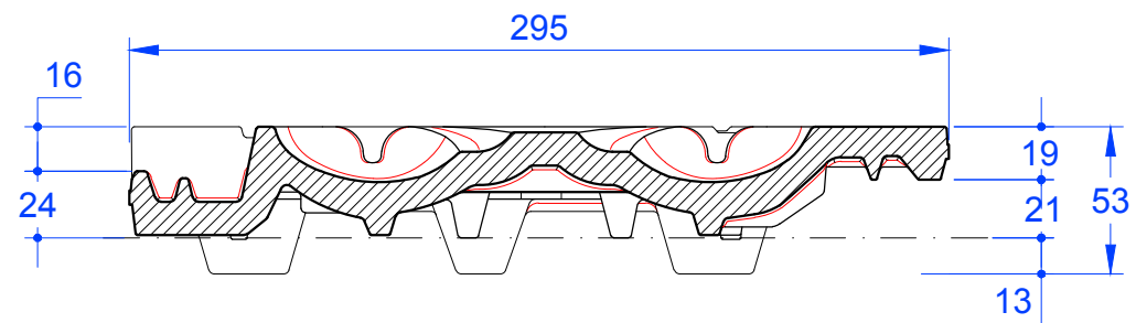
Schnitt A-A
