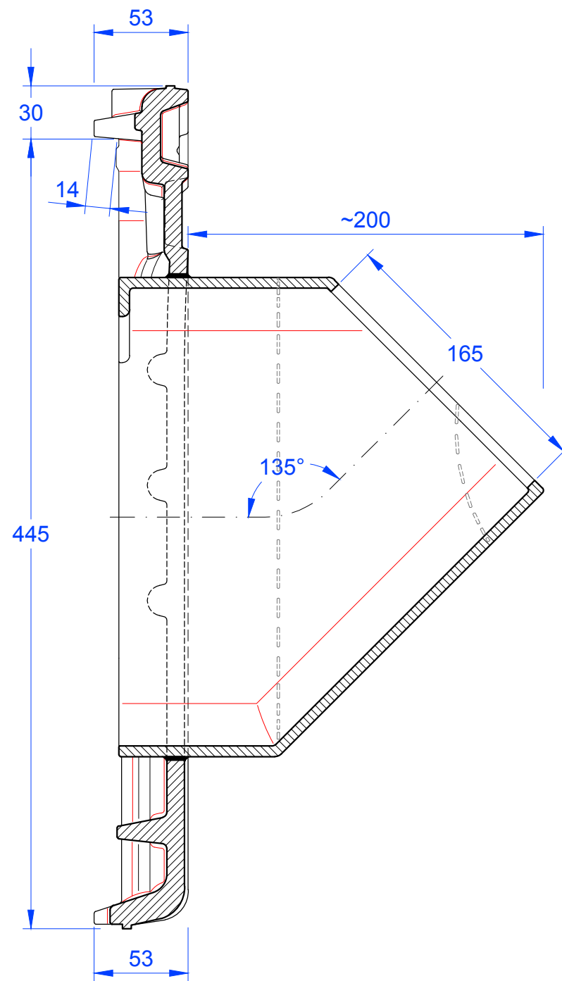
Schnitt B-B
