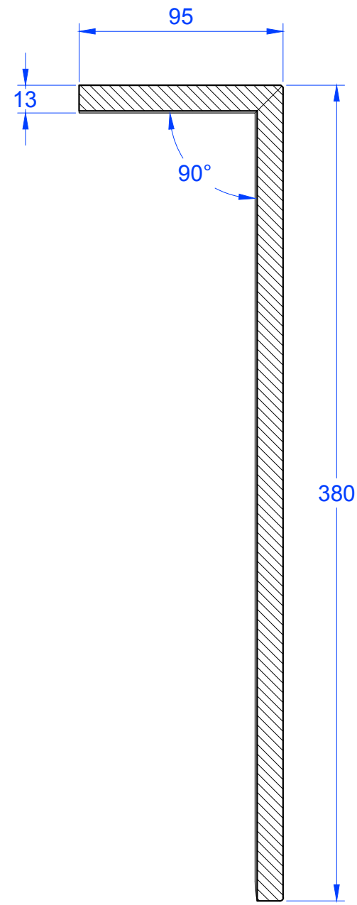
Schnitt B-B
