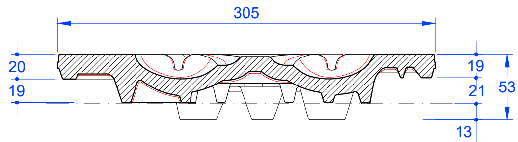
Schnitt A-A
