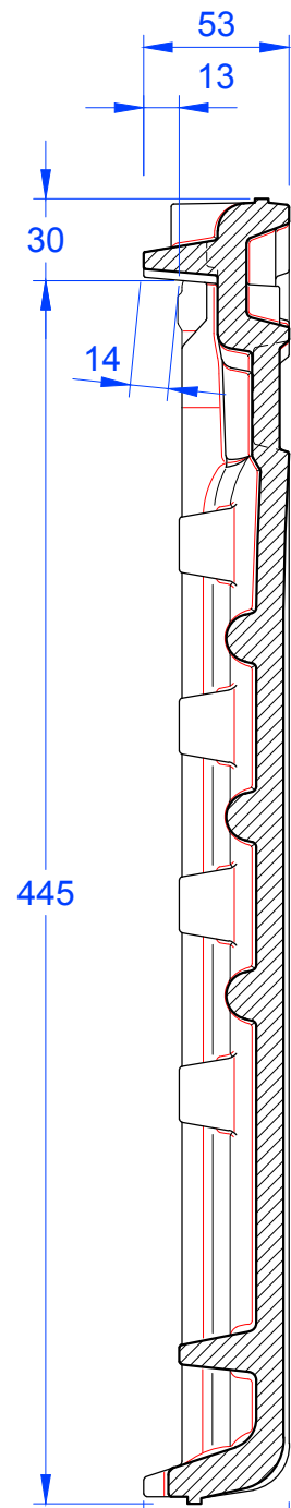
Schnitt B-B
