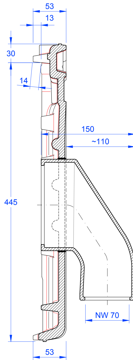
Schnitt B-B
