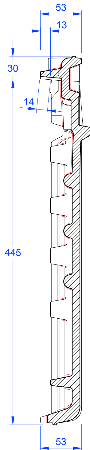
Schnitt B-B
