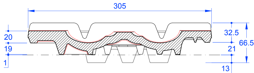
Schnitt A-A
