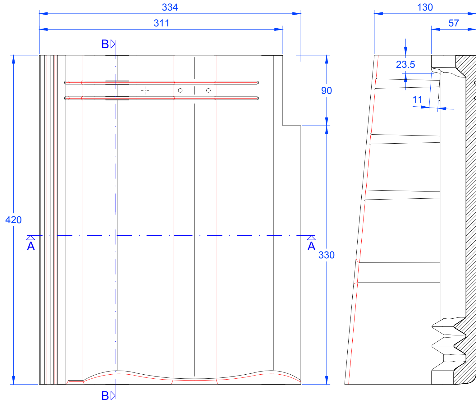
Schnitt B-B
